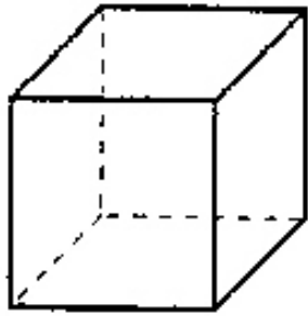
le cube
