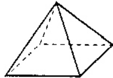
la pyramide
