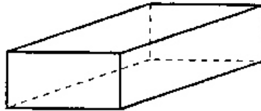
le prisme
