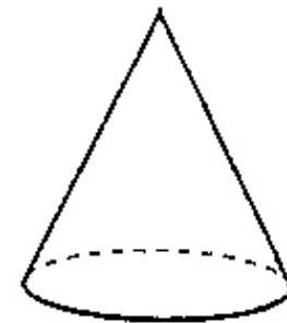
le cône
